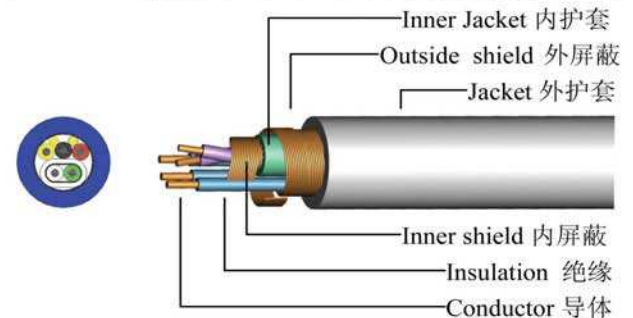
DX0009A ECG raw cable 五芯病人电缆
